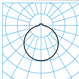
74R G2 WD3 DW 33-840 +HFS TX280829
