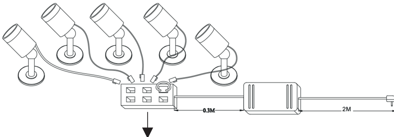
2 - Anschluss mit Anschluss Set (nicht im Lieferumfang) / Connection with connection set (not included in scope of delivery)
