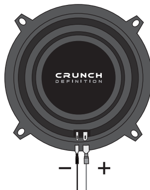
ANSCHLÜSSE FÜR DEN VERSTÄRKER RECHTER KANAL
