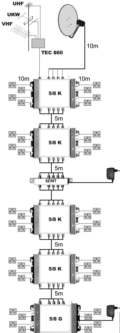
Pegelplan (Beispiel)
