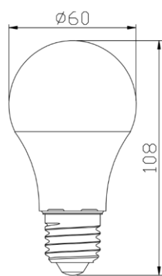
Abmessungsskizze LED MT65006
