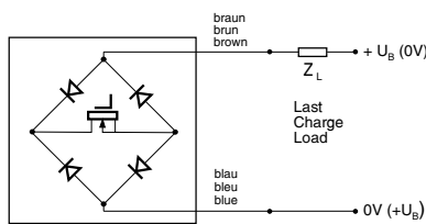
Kabelauführung / Version câble / Cable version
