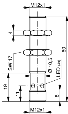
DW-AS-70x-M12-303
