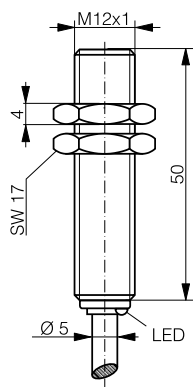
DW-AD-70x-M12-303
