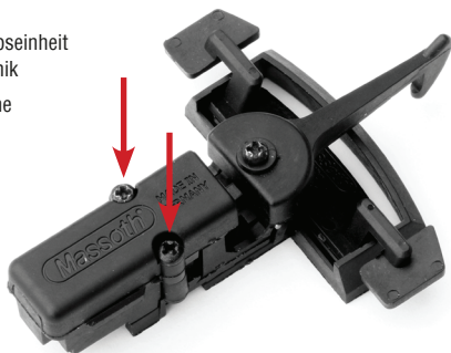
Abbildung 6: Montieren der Antriebseinheit an die Entkuppelmechanik Figure 6: Mount the drive unit to the uncoupler mechanism
