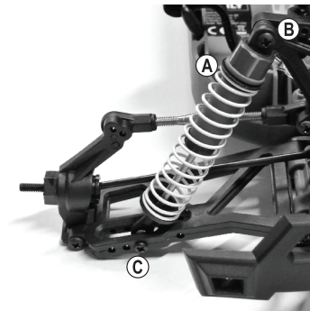
Vorderachse
