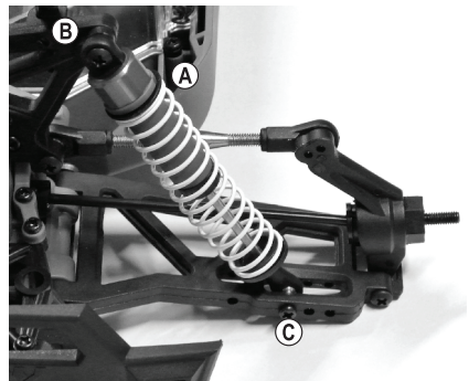
Hinterachse
