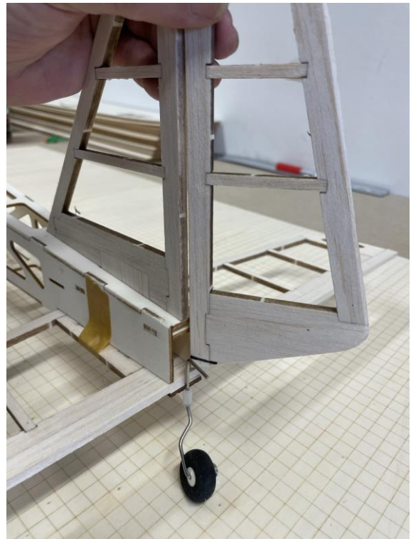
Seitenruder mittig bohren damit der abgewinkelte Fahrwerksdraht eingesteckt werden kann.
