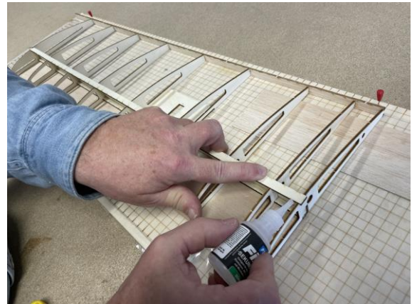
Obere Leiste B2 verkleben.
