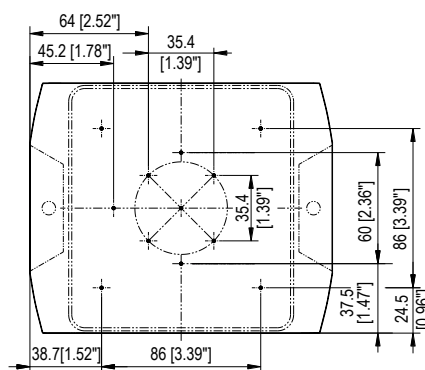
Схема расположения отверстий внутри корпуса
