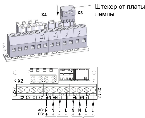
Подключение рабочего напряжения излучателя звука
