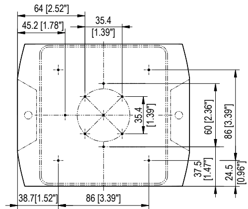
Schéma de perçage de l'intérieur du boîtier
