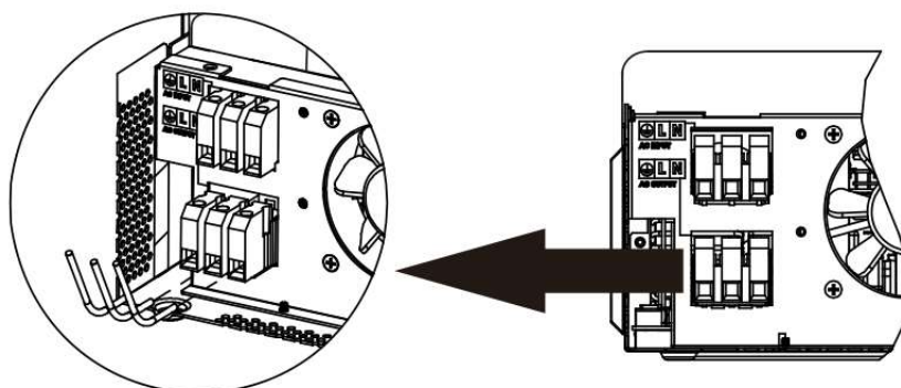
Abb. 8: AC-Ausgangsanschluss
