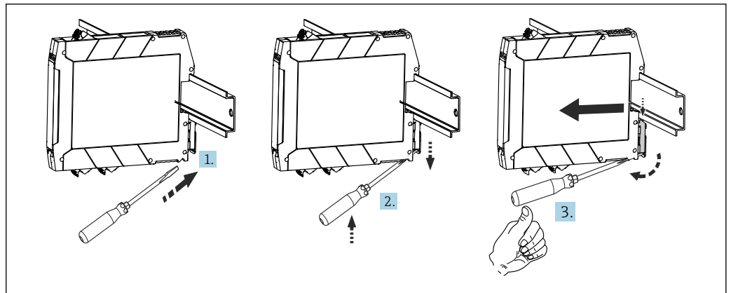
4 Hutschienengerät demontieren
