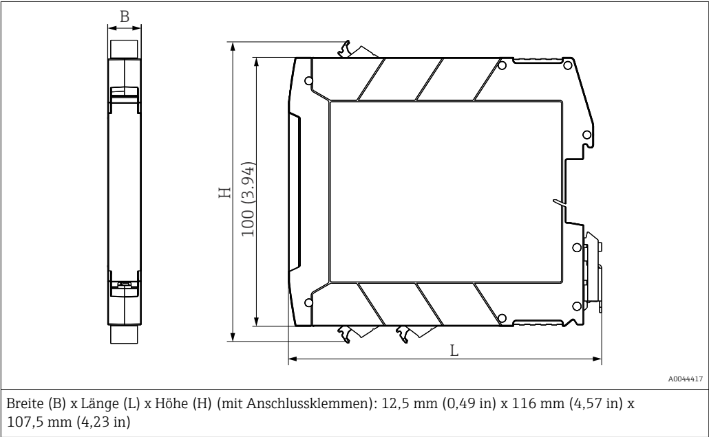
Klemmgehäuse zur Montage auf Hutschiene
