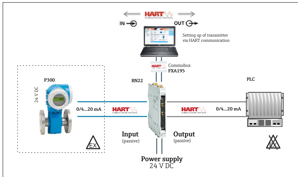
18 Durchflussmessung im explosionsgeschützten Bereich mit einem Speisetrenner RN22
