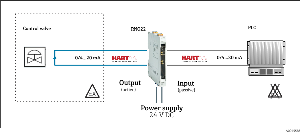
23 Regelventilansteuerung im Ex-Bereich mit einem Ausgangstrennverstärker RNO22
