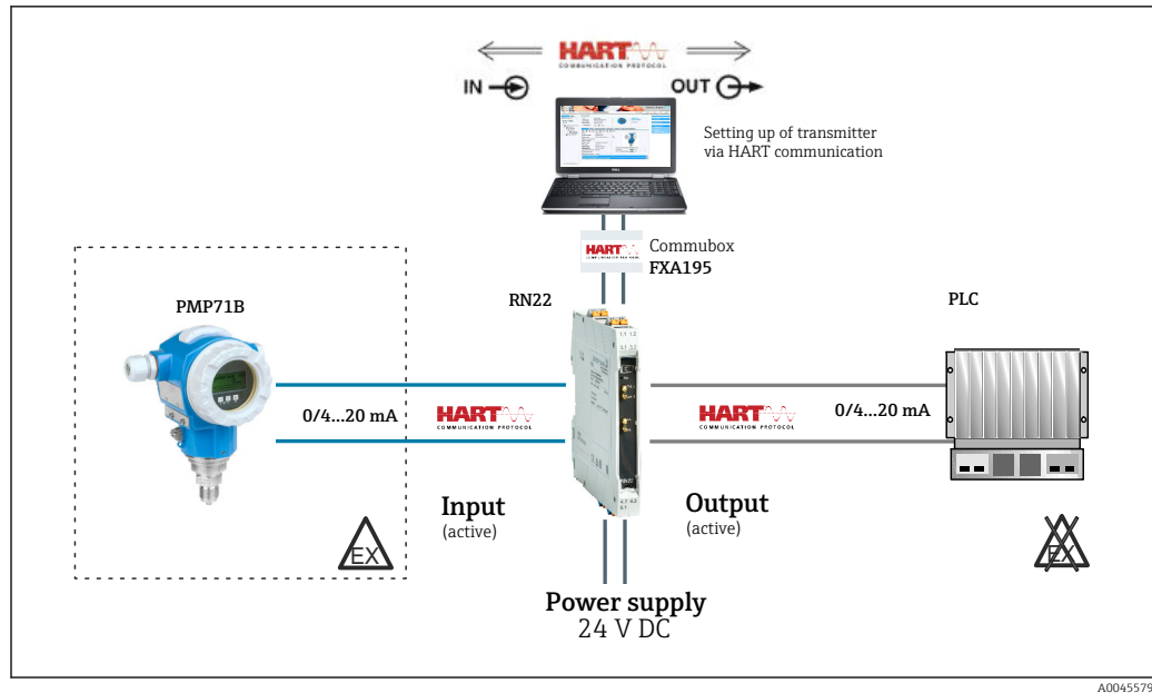
17 Druckmessung in einem explosionsgeschützten Bereich mit einem Speisetrenner RN22
