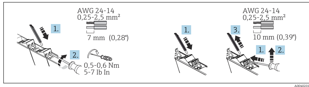
5 Elektrischer Anschluss mittels Schraubklemmen (links) und Push-in Anschlussklemmen (rechts)
