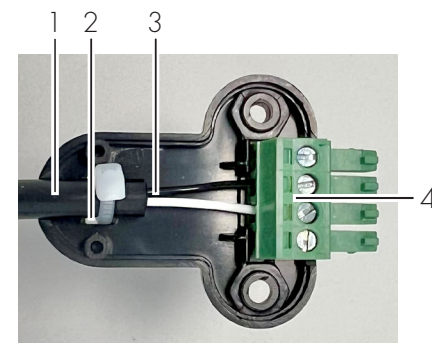
Bild 4 PT1000-Adapter
