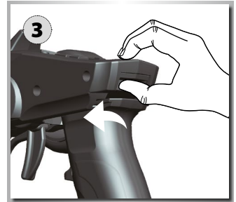
Handgriff installieren
