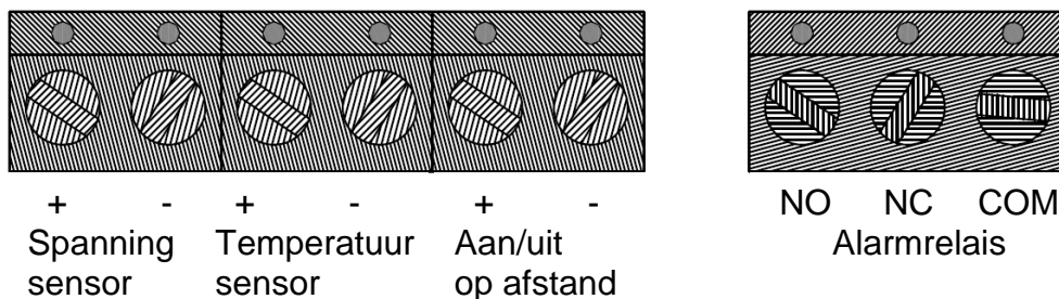
Afbeelding 5 Aansluitblok
