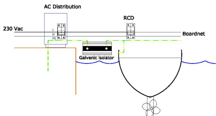
Abbildung 1: Schaltbild
