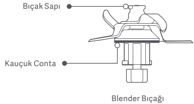
Blender Bıçađı
