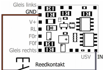
Fig. 6: Anschluss eines Reedkontaktes an den Schalteingang
