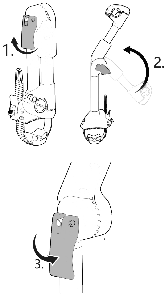
Figure 3 : Adaptation au diamètre de l'étrier en U
