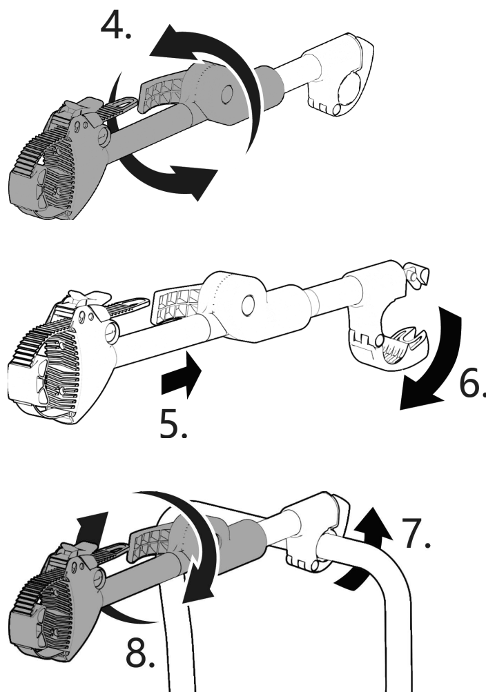
Bild 4: Montage an U-Bügel
