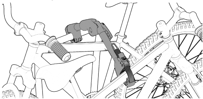
Bild 5: Fahrrad befestigen
