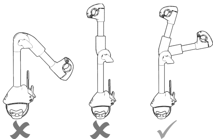
Figura 2: Ribaltamento del supporto del telaio
