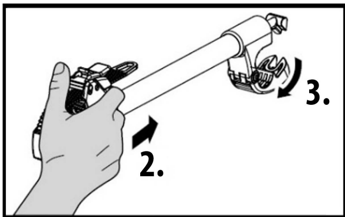
Bild 9: Rahmenhalter öffnen
