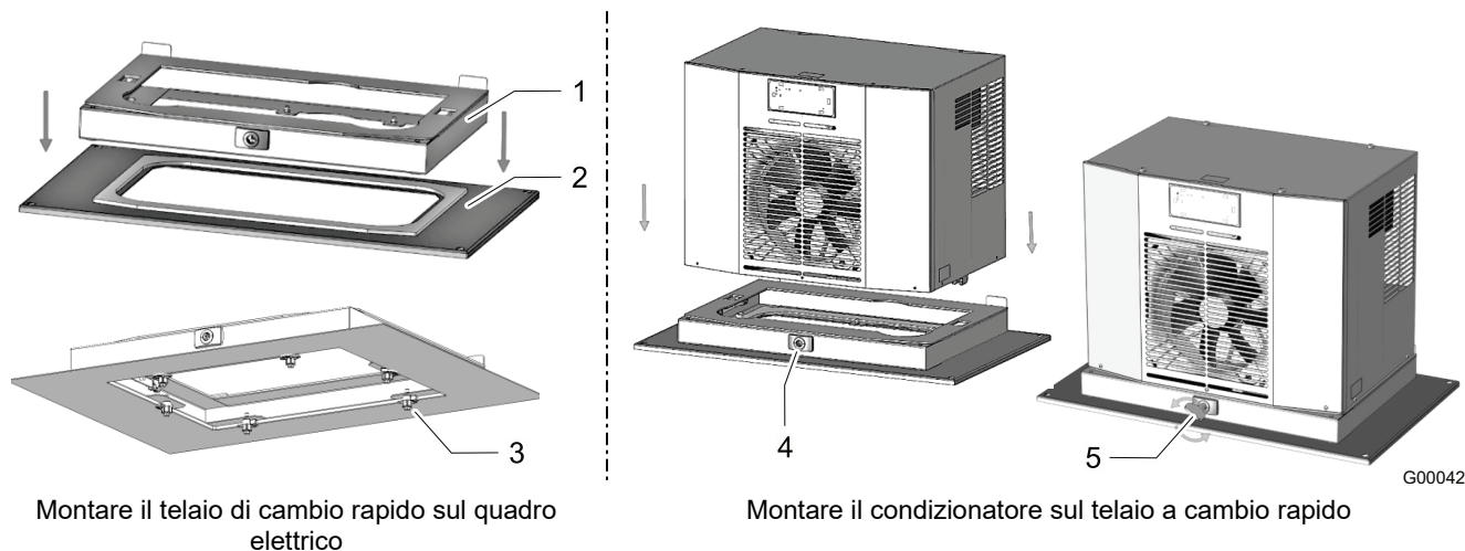
Fig. 21: Montare la staffa
