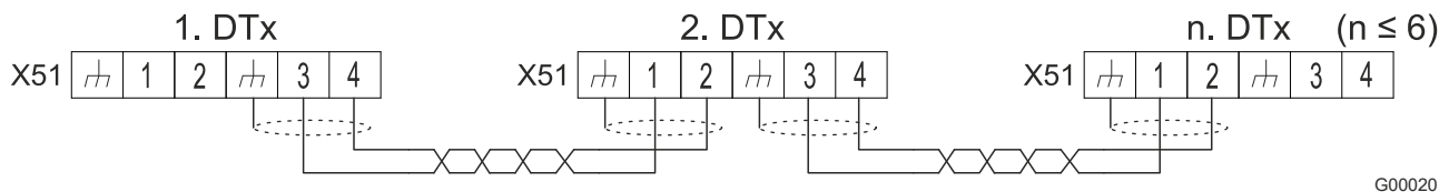
Рис. 23.: Мультимастерное управление
