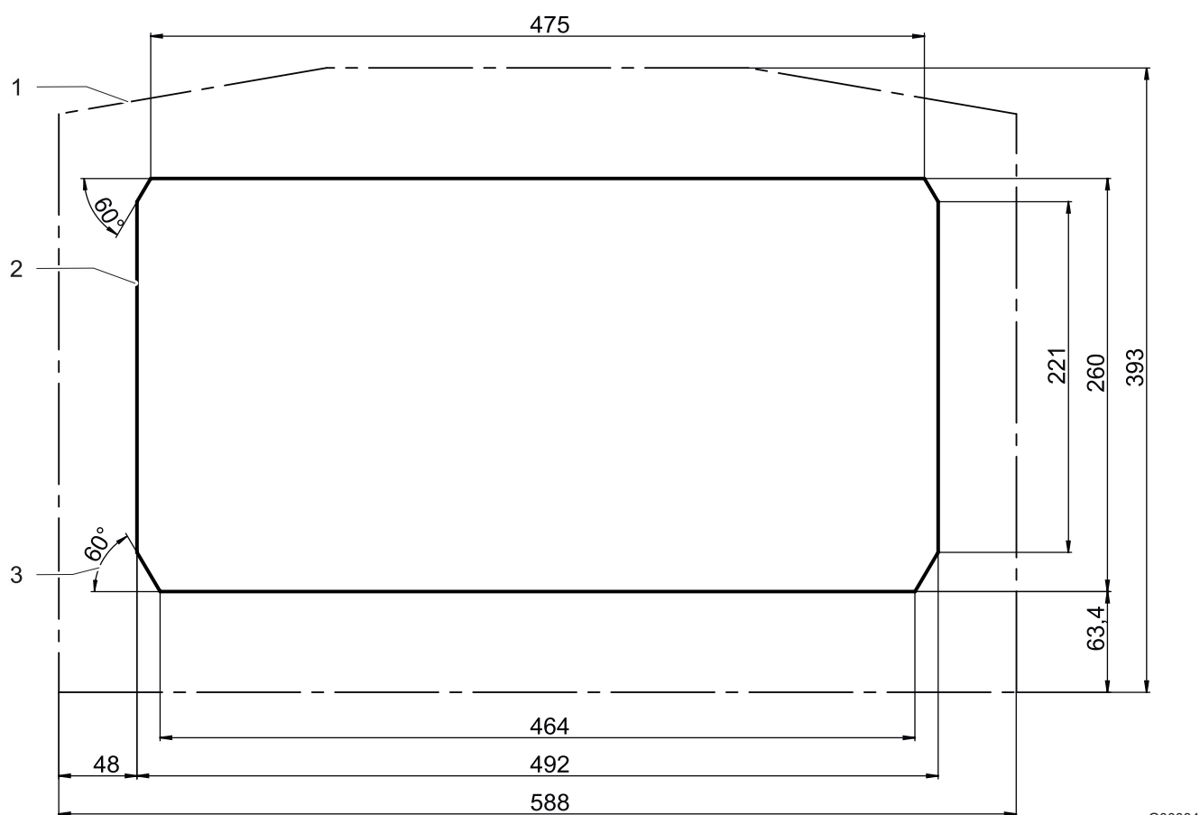
Fig. 14: Recorte del armario eléctrico «Easy Cut»
