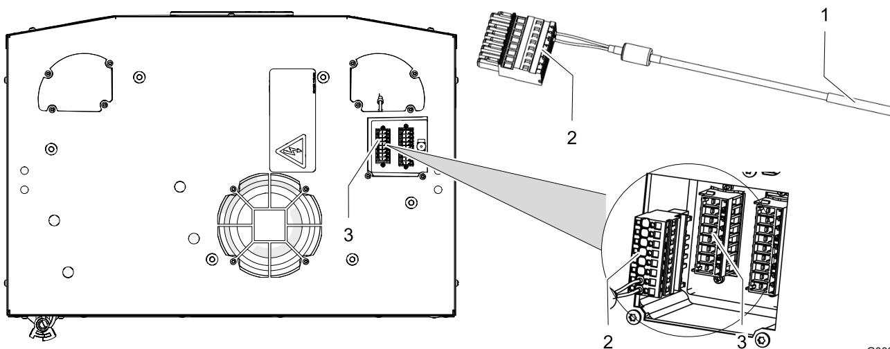
Fig. 24 : capteur de température – TS2
