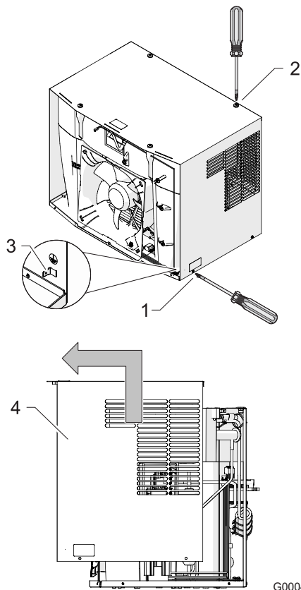
Abb. 19: Gerätehaube entfernen
