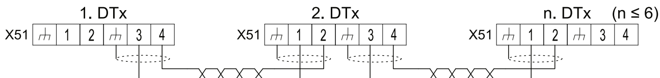
Fig. 11 : Commande multimaître
