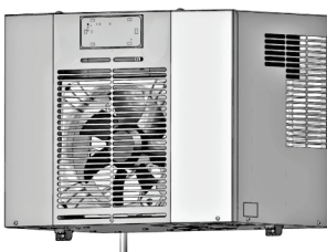
Fig. 20 : montage du support
