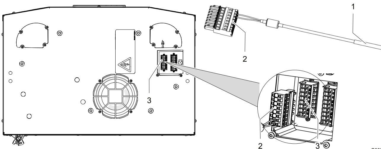
Fig. 10 : capteur de température – TS2
