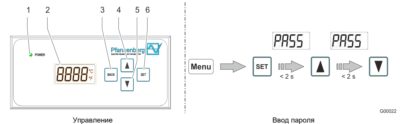
Рис. 27.: Блок управления мультиконтроллера (MC)
