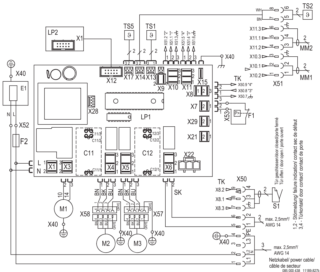
Fig. 22 : schéma de câblage
