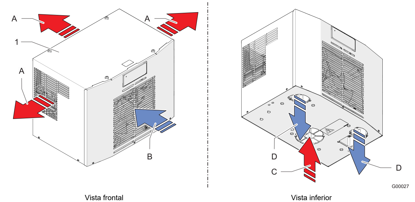
Fig. 1: Circuito de aire del armario eléctrico DTT
