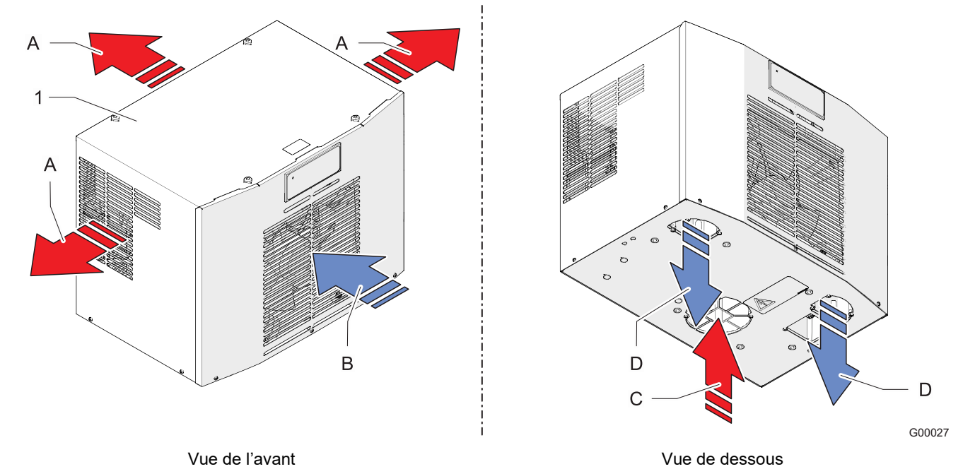
Fig. 1 : circuit d'air de l'armoire de distribution DTT
