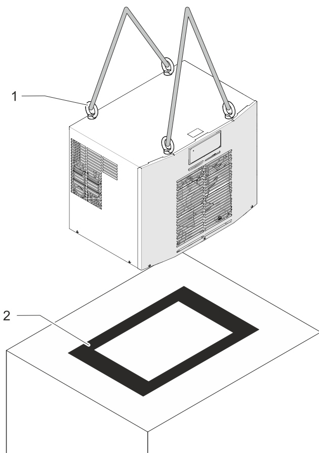
Рис. 17.: Монтаж устройства охлаждения с завертками
