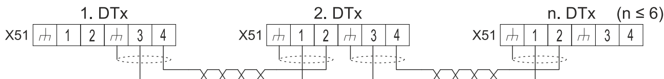
Рис. 11: Мультимастерное управление
