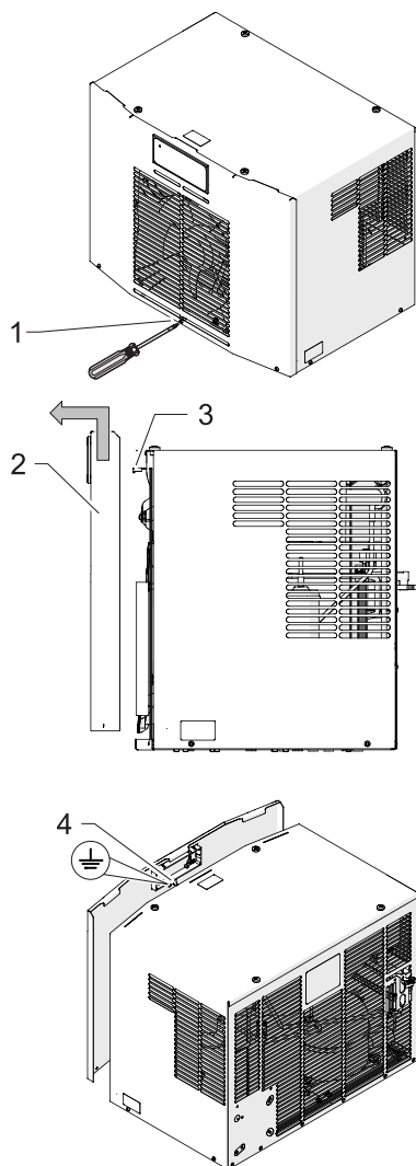
Abb. 30: Frontklappe demontieren
