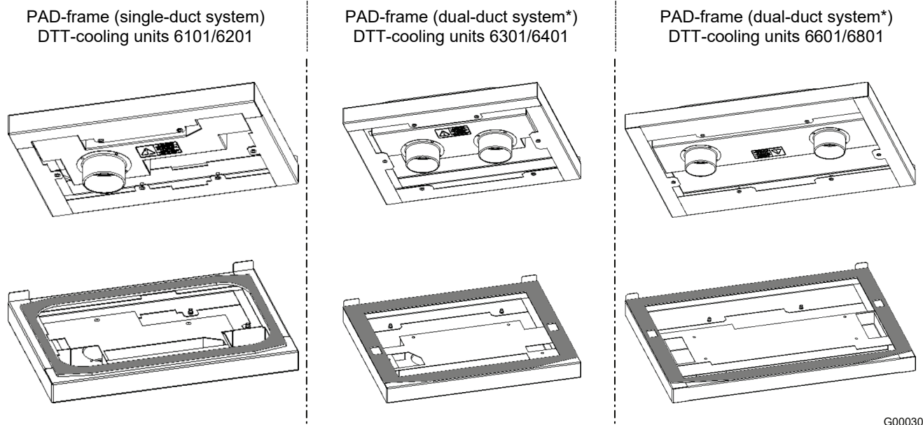
Fig. 5: PAD-frame
