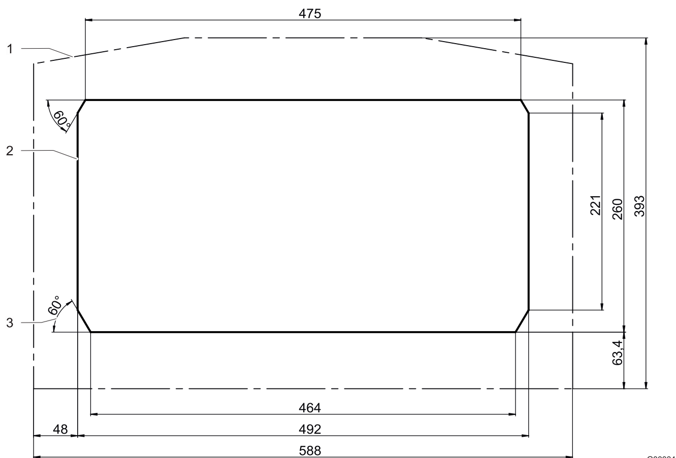
Fig. 14: découpe « Easy-Cut » de l'armoire de distribution
