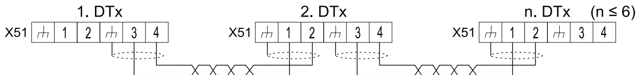
Abb. 11: Multimaster-Steuerung
