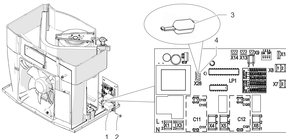
Рис. 28.: Сервисный интерфейс
