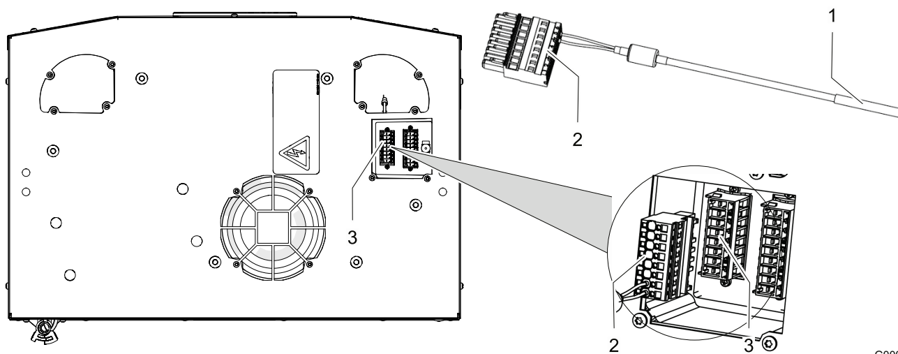
Abb. 10: Temperatursensor - TS2
