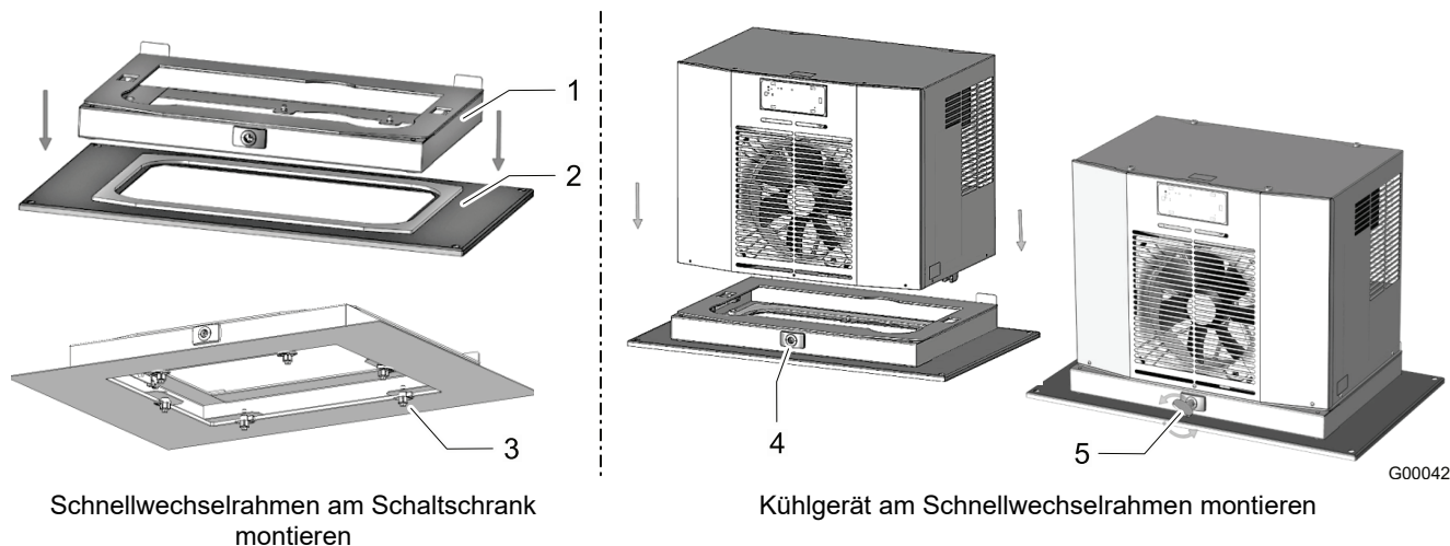
Abb. 21: Halterung montieren
