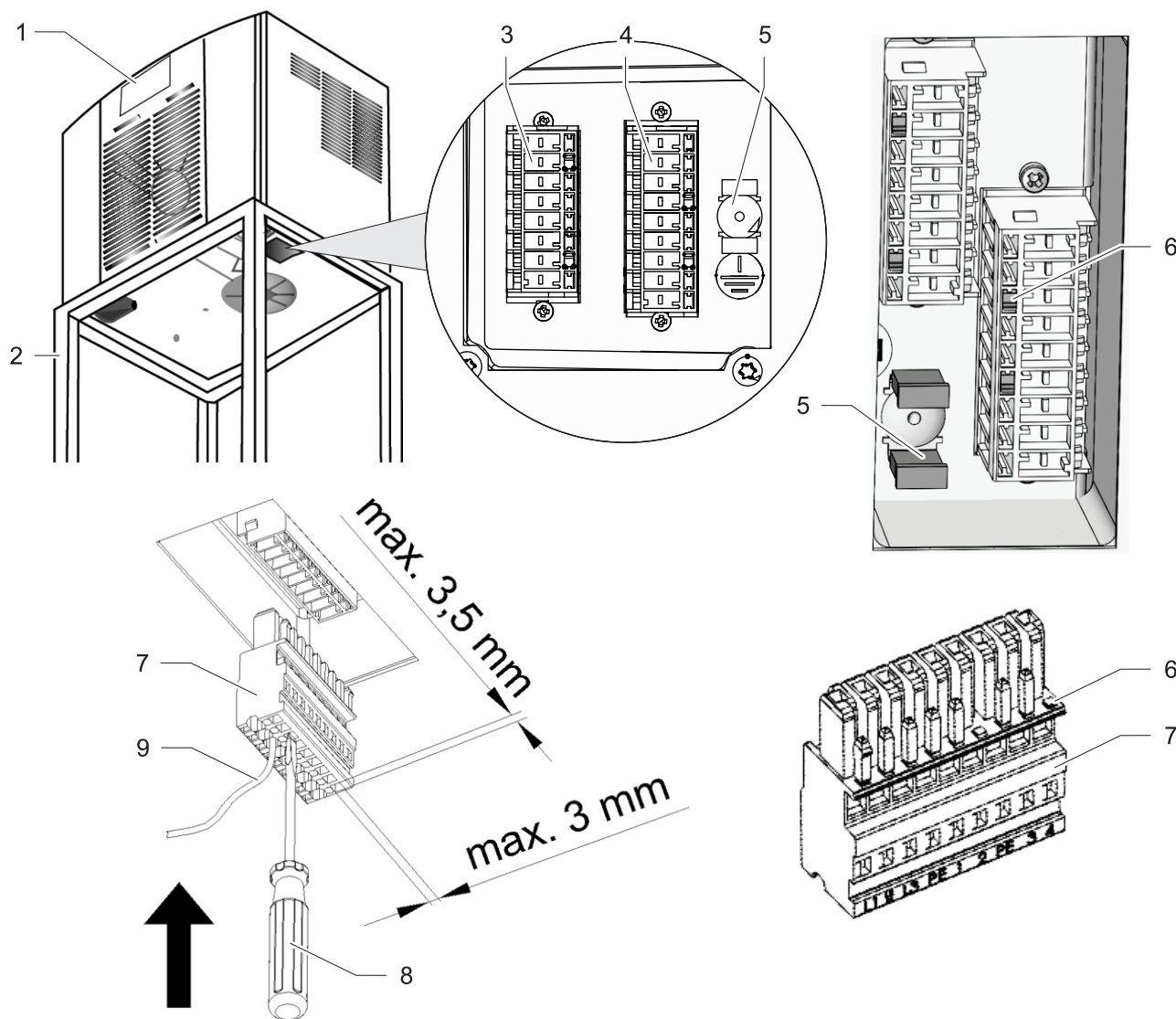
Abb. 25: Netz-Anschlussstecker Kühlgerät
