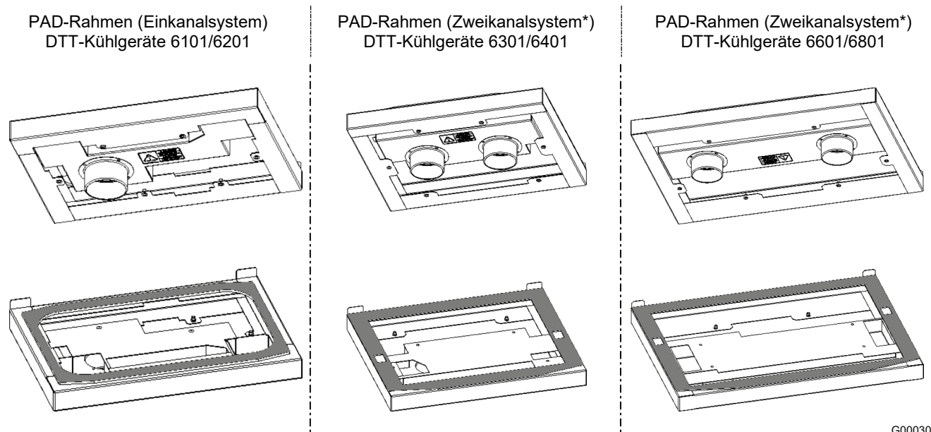
Abb. 5: PAD-Rahmen
