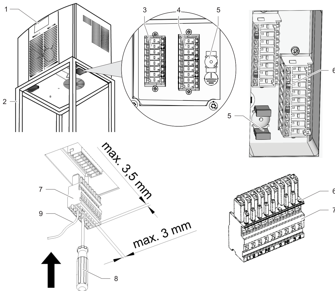
Fig. 25: Connettore di collegamento alla rete del condizionatore
