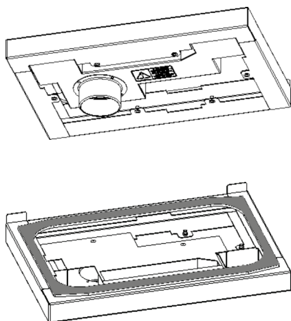
Fig. 5: Châssis PAD
