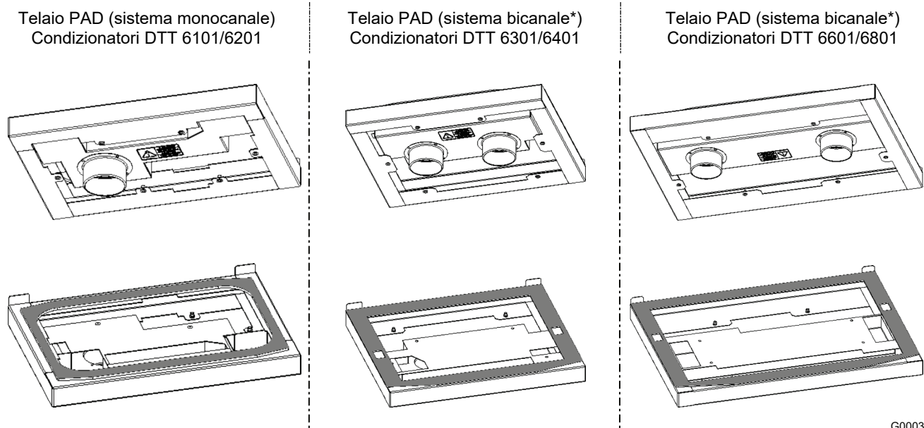
Fig.5: Telaio PAD
