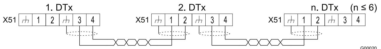
Abb. 23: Multimaster-Steuerung
