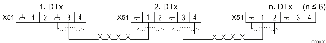
Fig. 23: Commande multimaître
