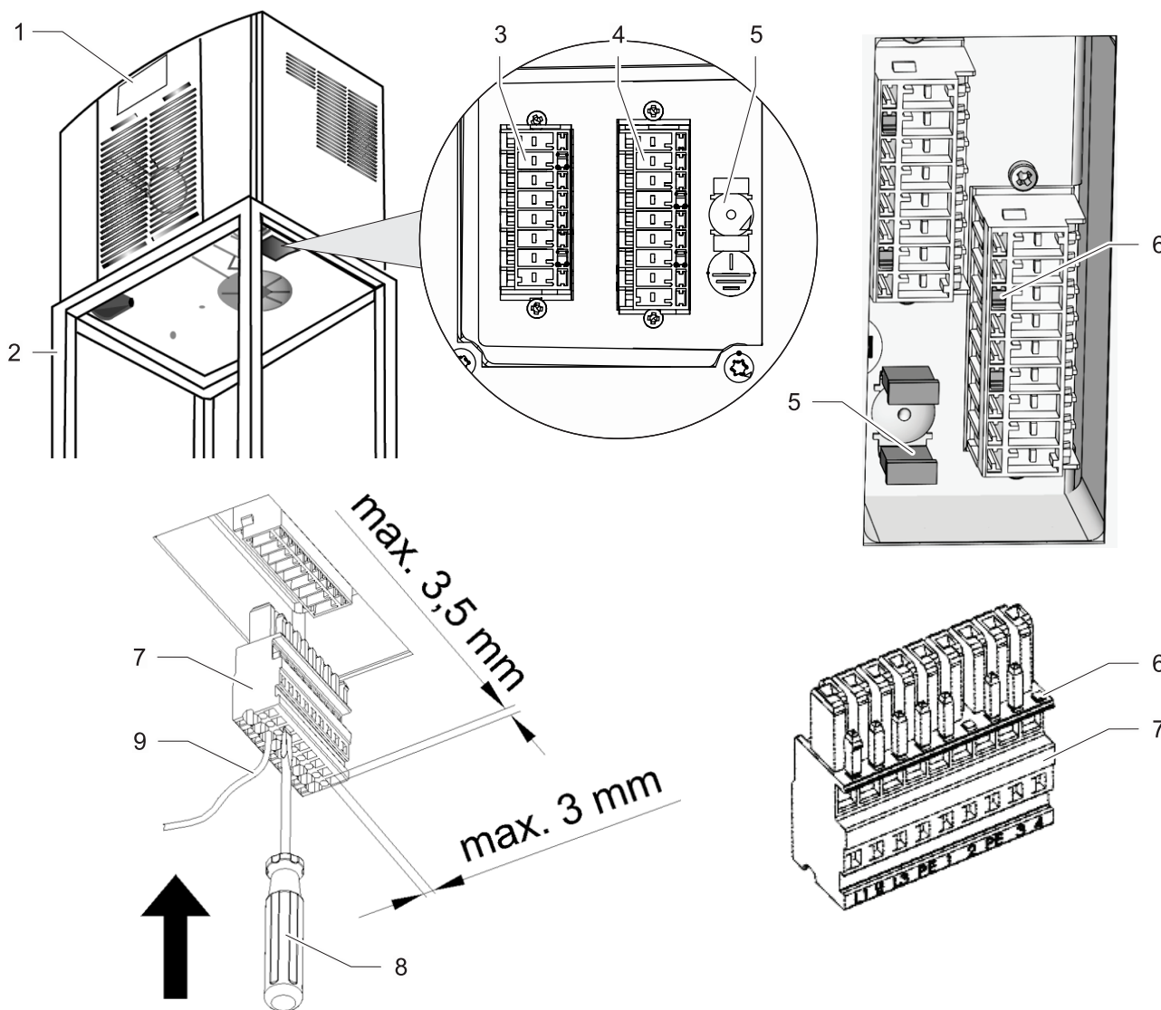
Fig. 25 : fiche de raccordement secteur du climatiseur
