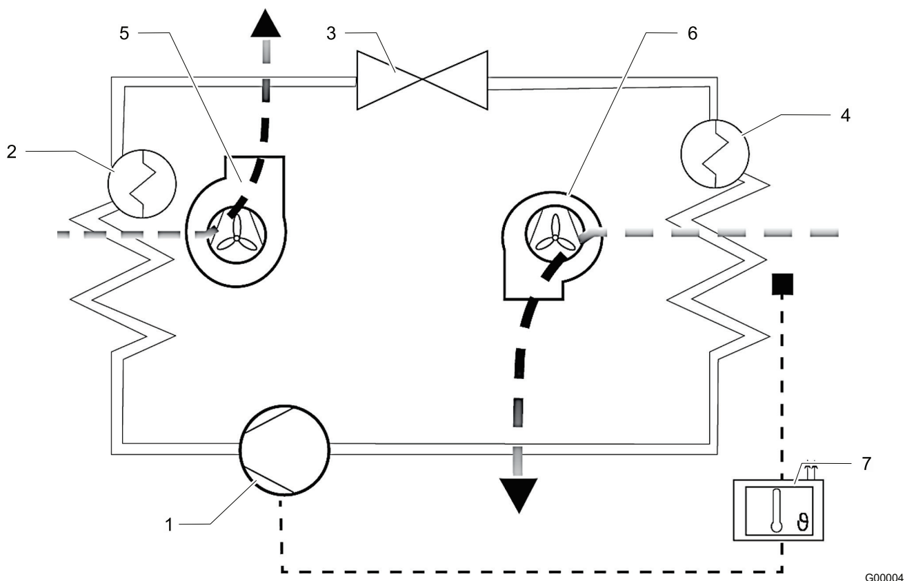
Abb. 7: Kältekreislauf
