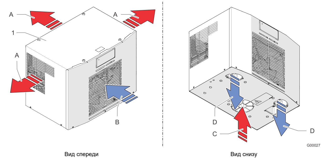
Рис. 1: Циркуляция воздуха в шкафу управления DTT
