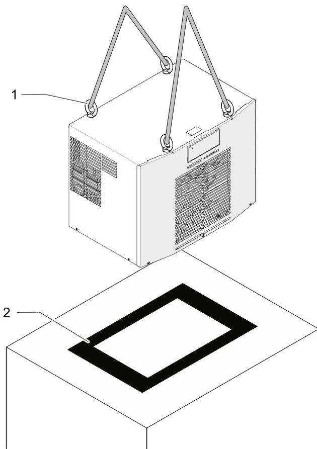
Fig.17: Montaggio del condizionatore con dispositivi di fermo
