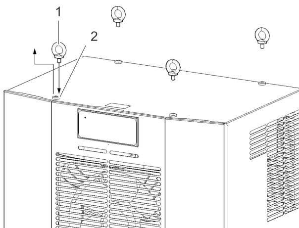
Рис. 13: Подъемные проушины M8 устройств охлаждения DTT
