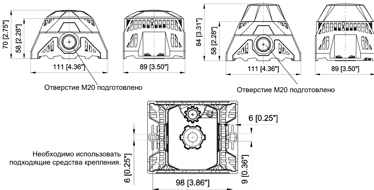
Схема расположения отверстий; вид снизу
