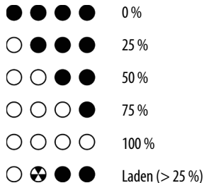
Bild 3: Ladezustandsanzeige
