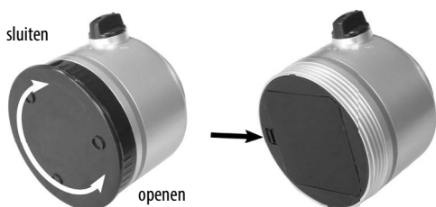
Afb. 2: Batterijvak openen
