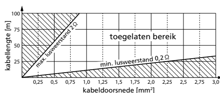
Afb. 5 Vereiste kabeldoorsnede voor de inductielus
