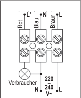
Schaltplan
