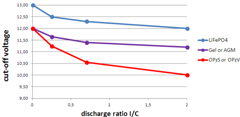
Entladeverhältnis in Abhängigkeit von der Batteriespannung für unterschiedliche Batterietypen
