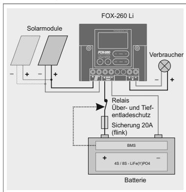
Diagramm: 1-Kanal Schutz
