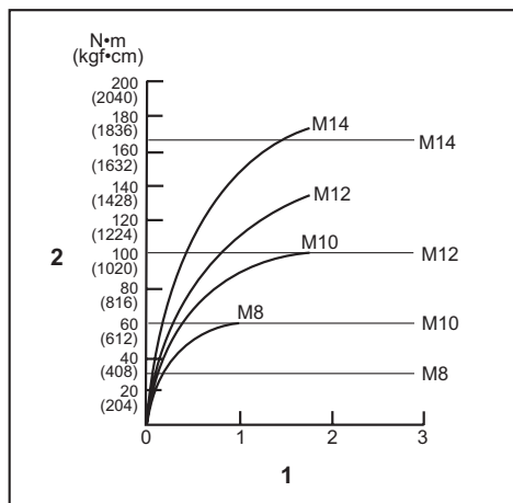
1. Aandratijd (seconden) 2. Aandratimoment
