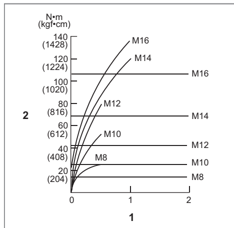
1. Aandratijd (seconden) 2. Aandratimoment
