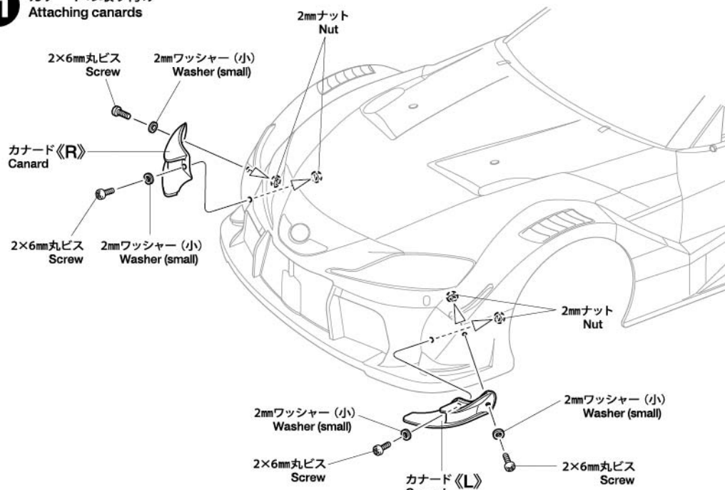
カナードの取り付け Attaching canards
