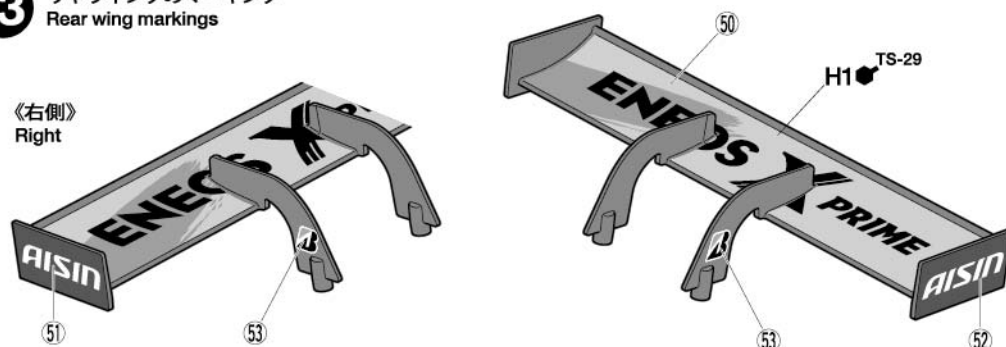
リヤウイングのマーキング Rear wing markings
