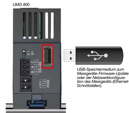
Abb. Messgerät - Ansicht von unten
