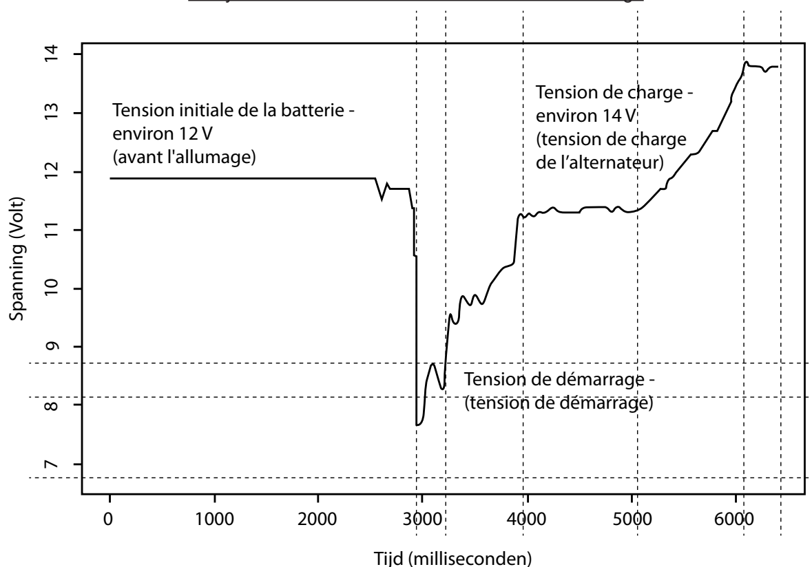
Analyse de la tension d'un véhicule lors d'un démarrage
