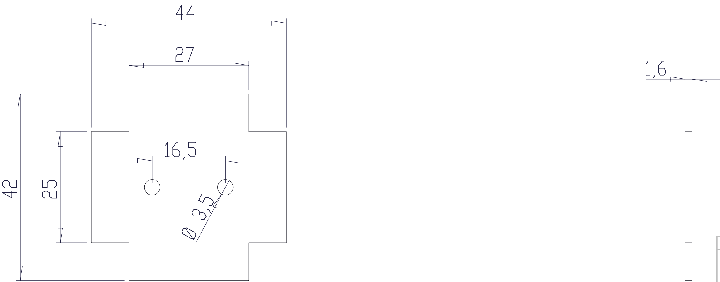
MUESTRA PCB
