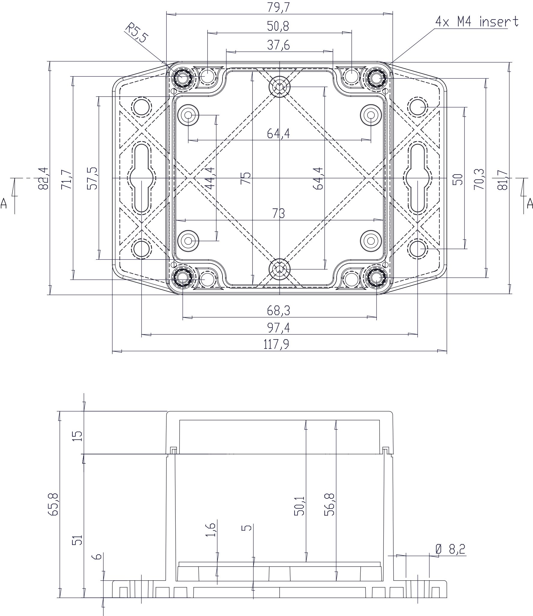
A-A
