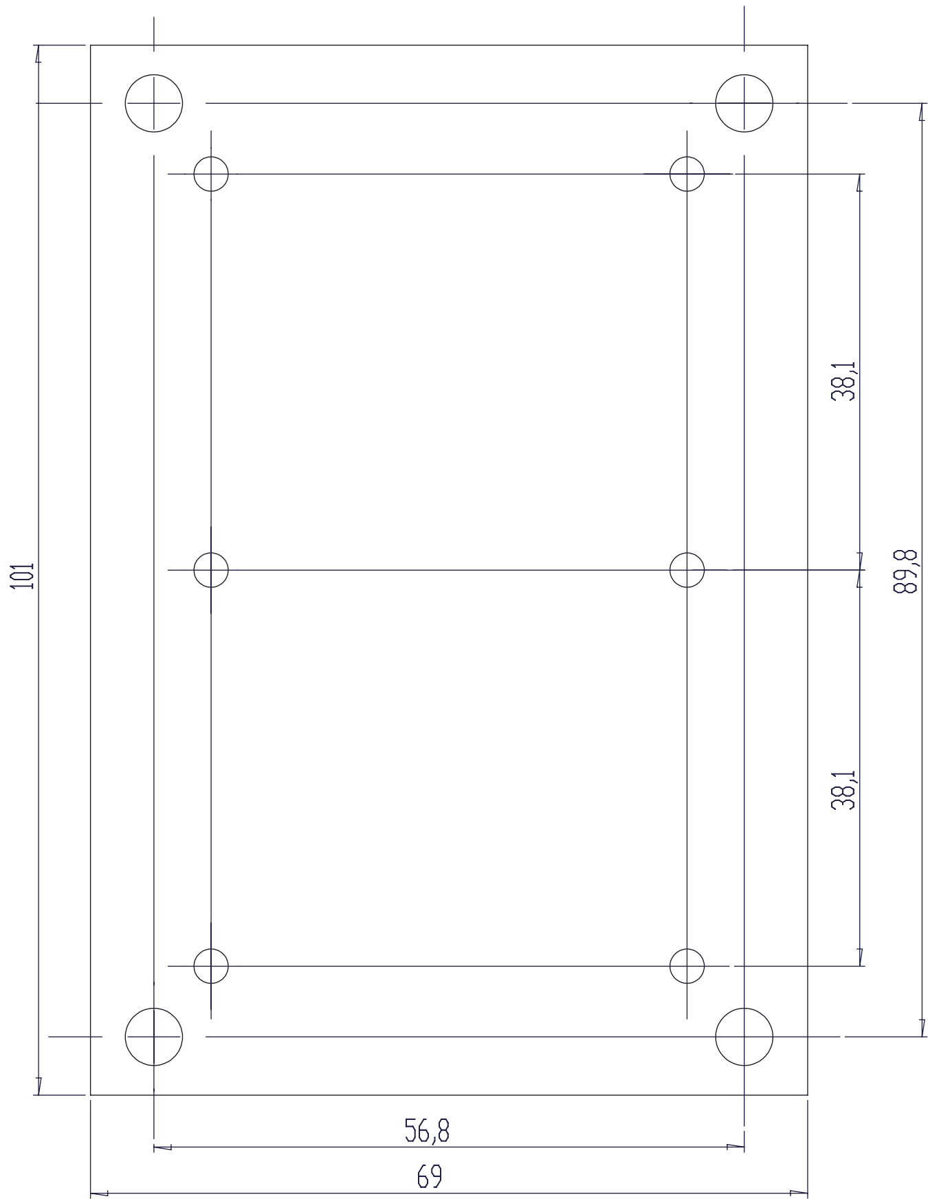
MUESTRA PCB
