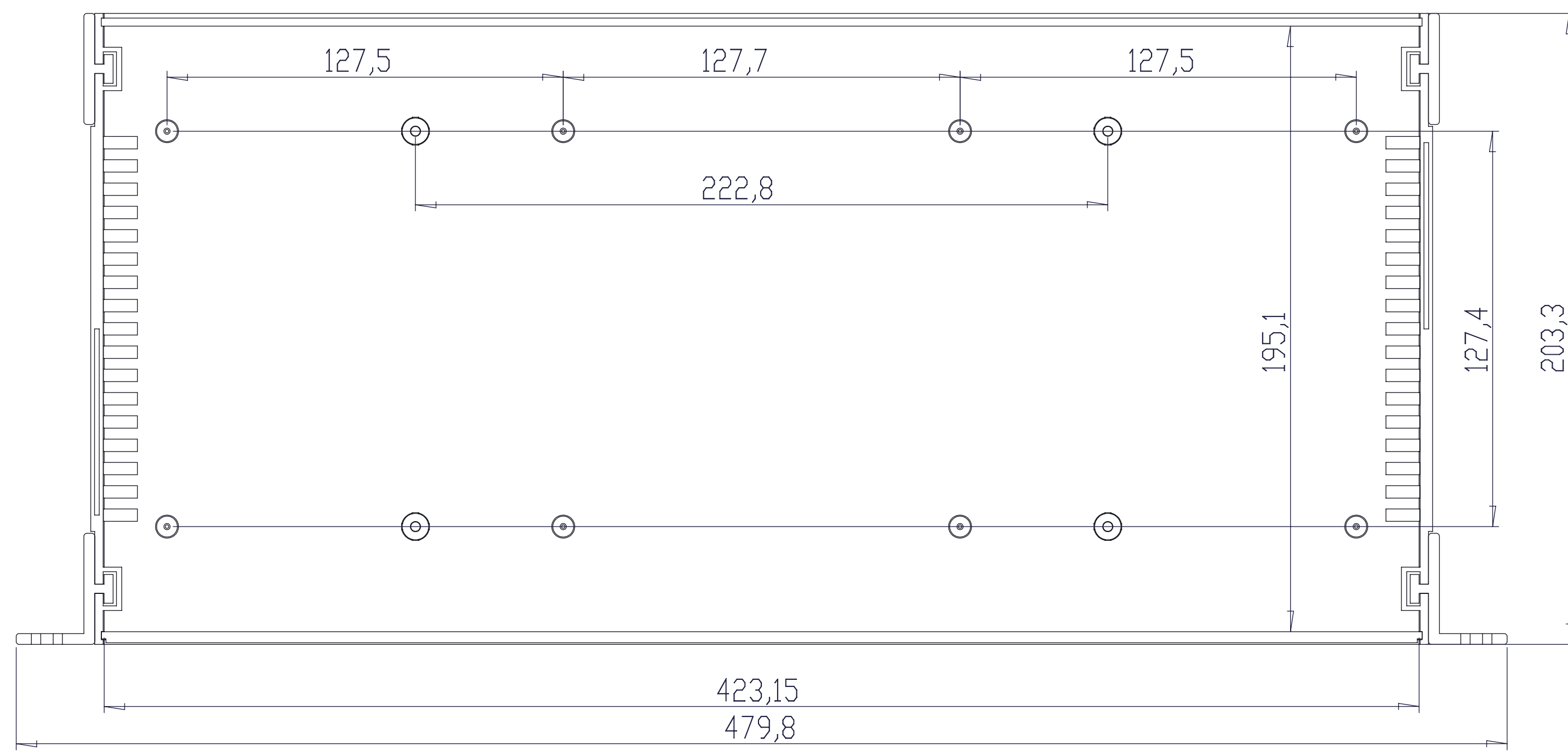
A-A
