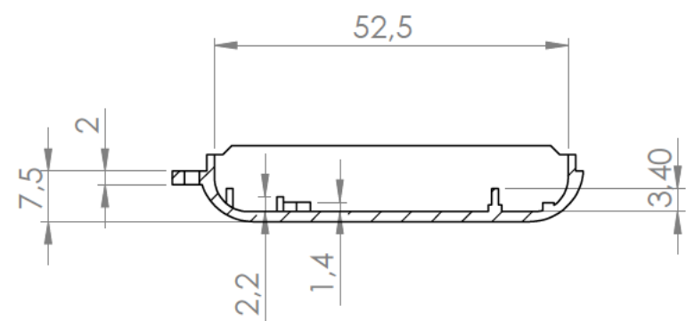
Sección/Section S-S
