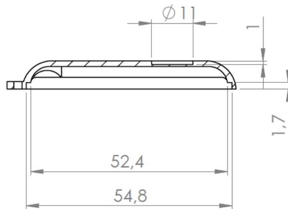
Sección/Section T-T
