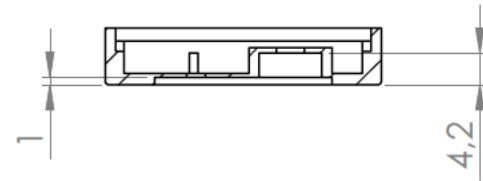
Sección/Section O-O
