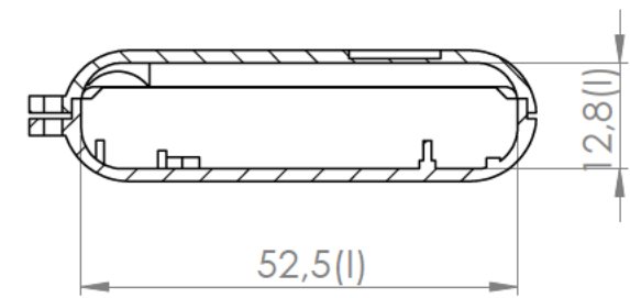
Sección/Section Q-Q
