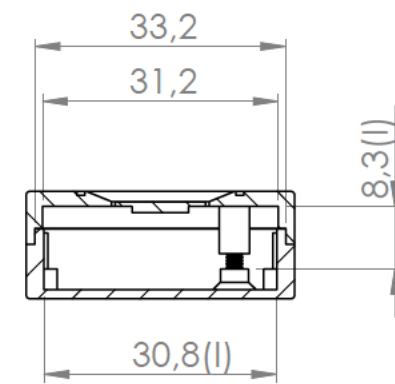
Sección/Section P-P
