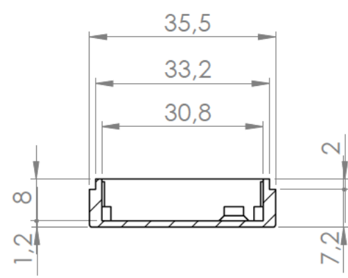
Sección/Section R-R
