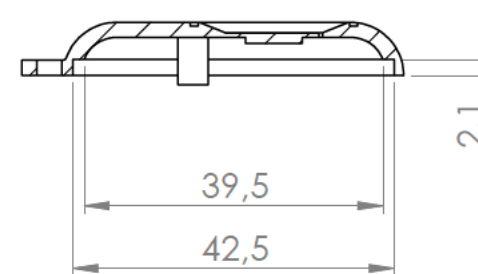
Sección/Section T-T
