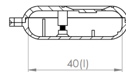
Sección/Section Q-Q
