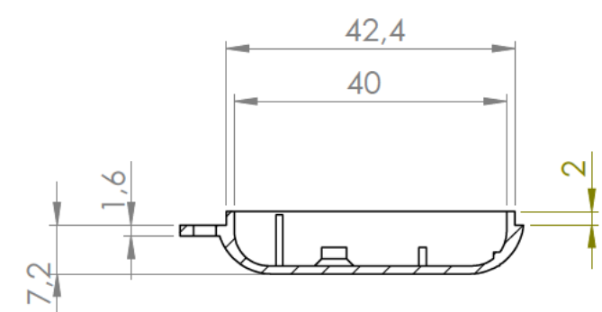
Sección/Section S-S
