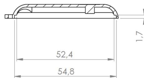
Sección/Section T-T
