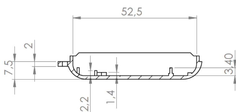
Sección/Section S-S
