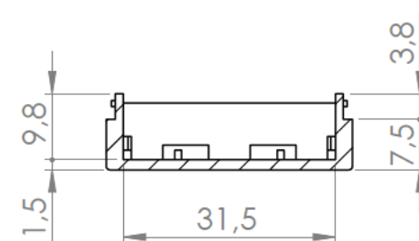
Sección/Section R-R
