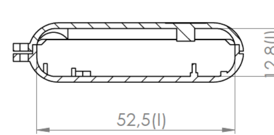
Sección/Section Q-Q
