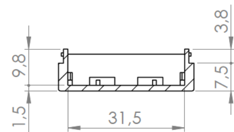
Sección/Section R-R
