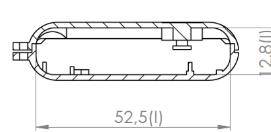
Sección/Section Q-Q
