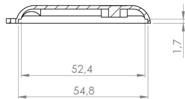
Sección/Section T-T
