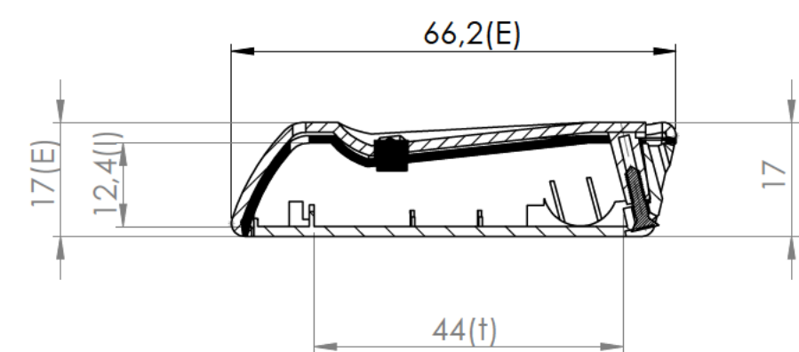
Sección / Section O-O
