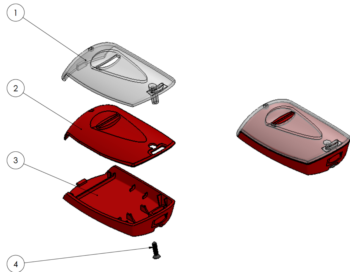
Conjunto Assembly
