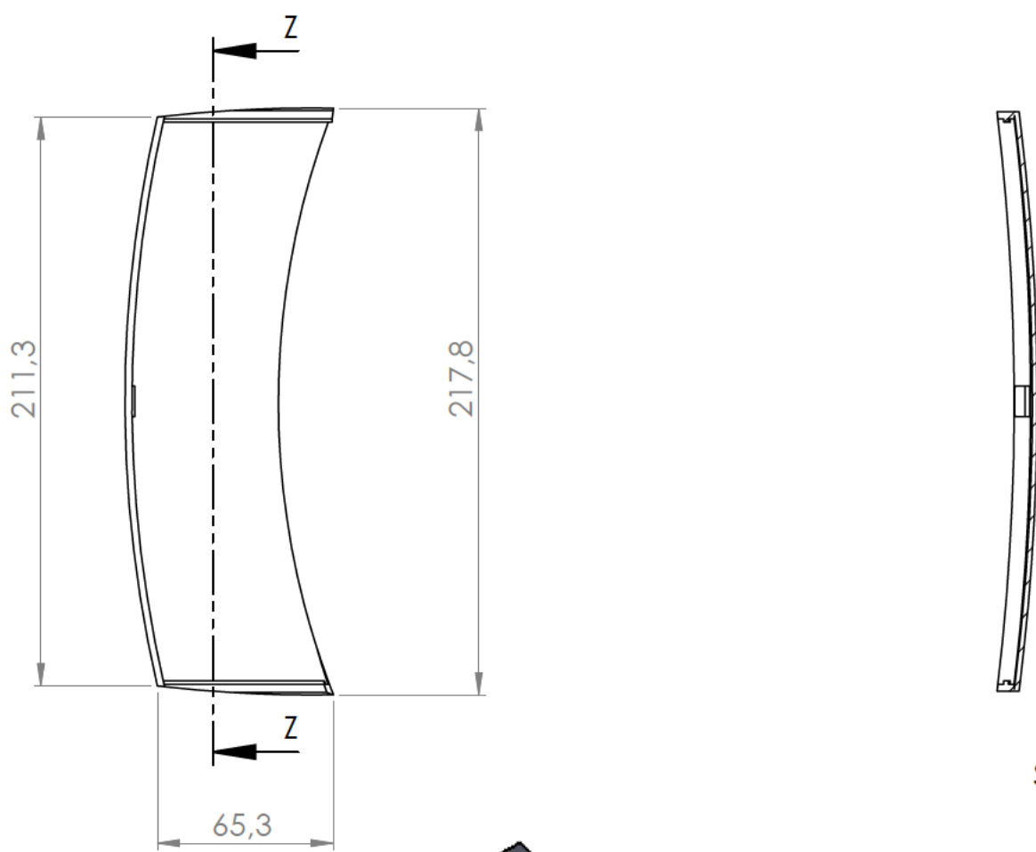
Sección / Section Z-Z
