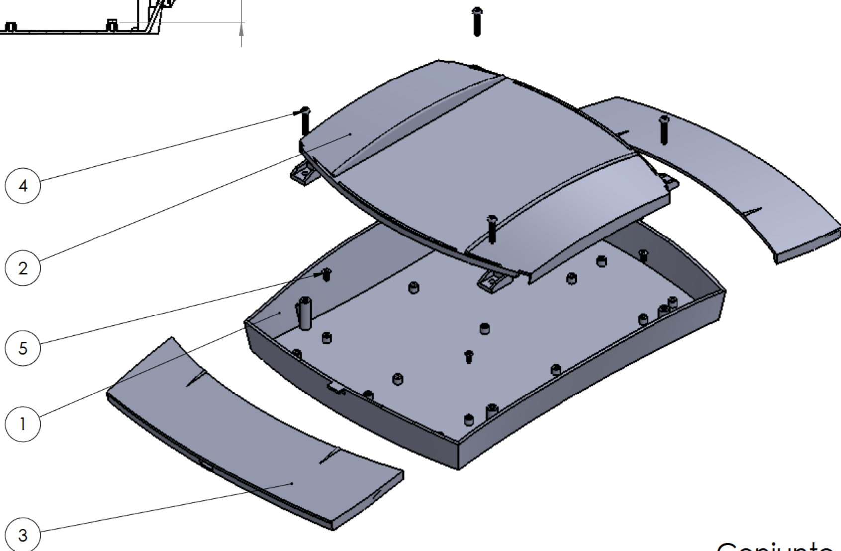
Conjunto Assembly
