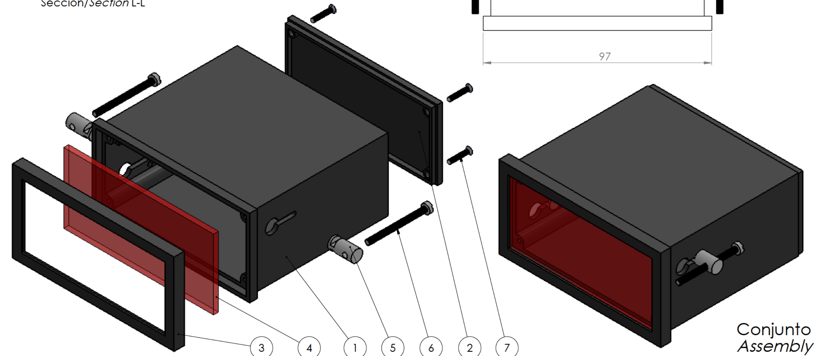
Sección/Section L-L
