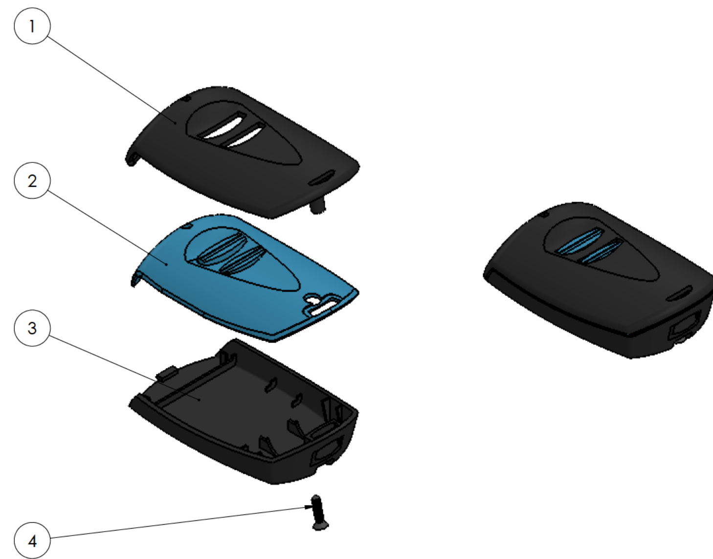
Conjunto Assembly
