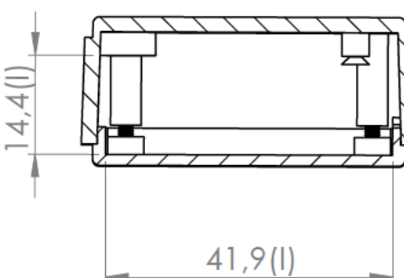
Sección /Section O-O
