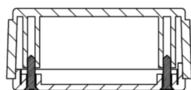
Sección / Section Q-Q
