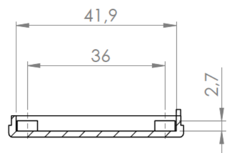
Sección /Section M-M
