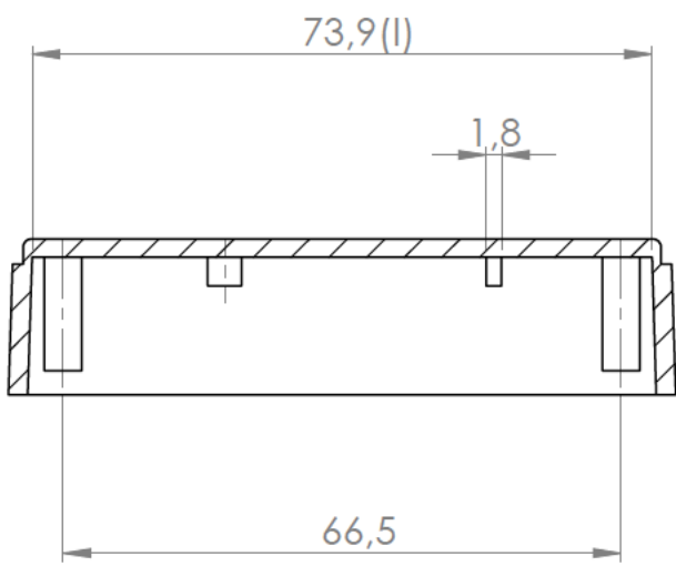
Sección /Section L-L
