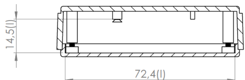
Sección /Section P-P
