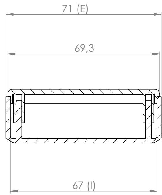
Sección/Section B-B
