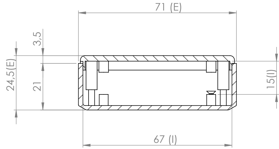
Sección G-G / Section G-G
