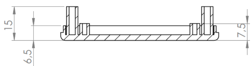
Sección J-J / Section J-J
