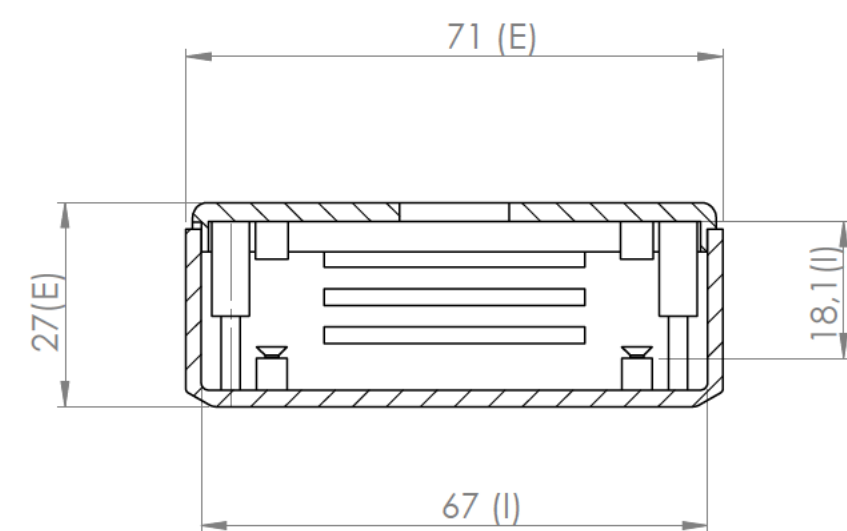
Sección G-G / Section G-G
