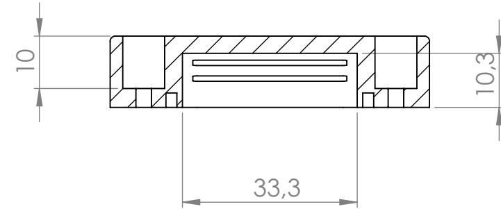
Sección/Section L-L
