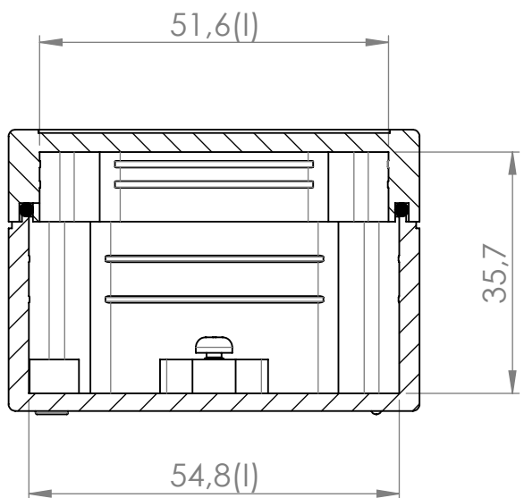
Sección/Section Q-Q
