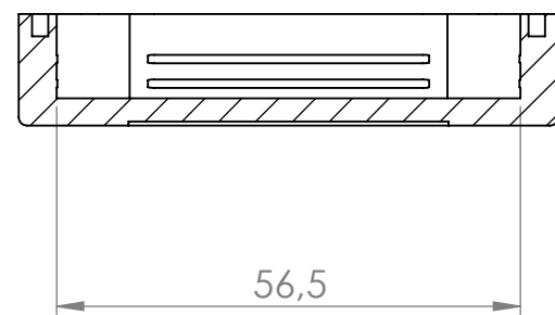
Sección/Section M-M
