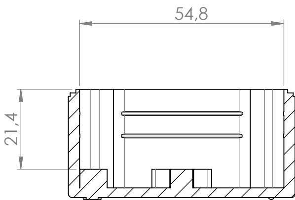
Sección/Section S-S
