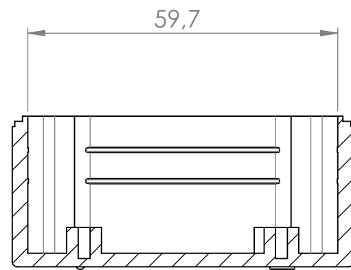
Sección/Section T-T
