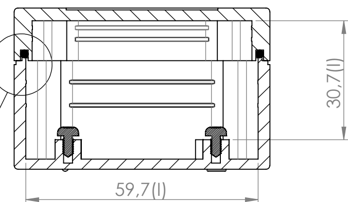
Sección/Section P-P
