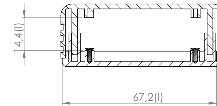
Sección / Section O-O
